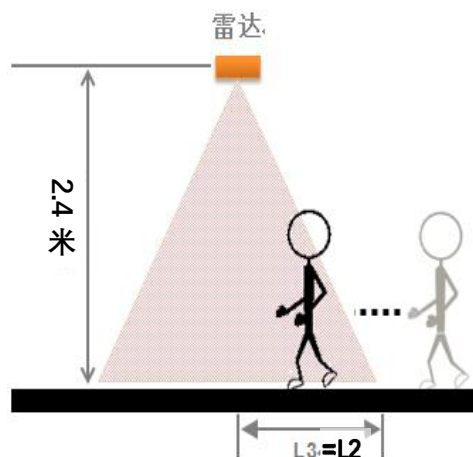
图 4 置顶安装示意图
