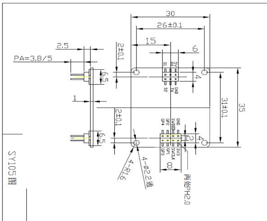
图1 雷达模块结构示意图
