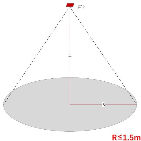
图 3 雷达波束覆盖范围示意图
