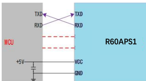
使用接线图
