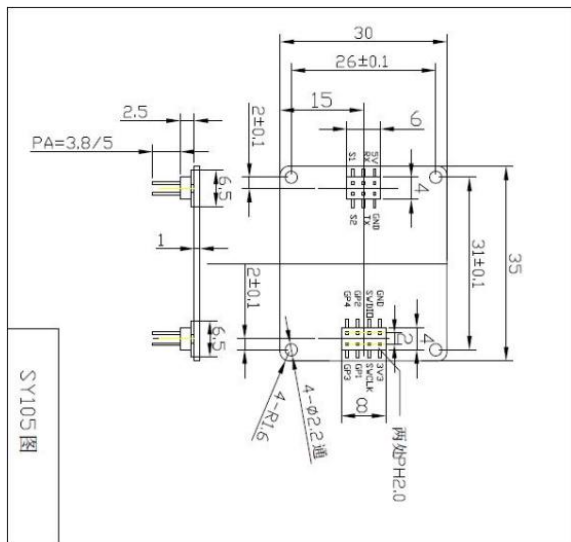
雷达模块结构示意图
